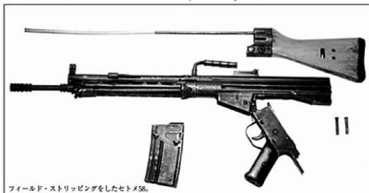
フィールド・ストリップングをしたセトメ58。
