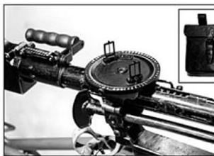
ダイヤル・サイトを装着したマドセン機関銃。ダイヤル・サイトは銃本体に付けるのではなく、三脚の一部(後部)を固定するクラップに装着します。
